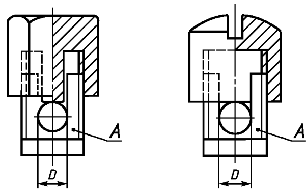
A — закрепленная часть; D — пространство для провода
