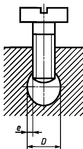
Зажим без прижимной пластины
