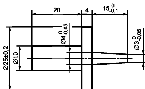
Рисунок 1 — Испытательный стержень
