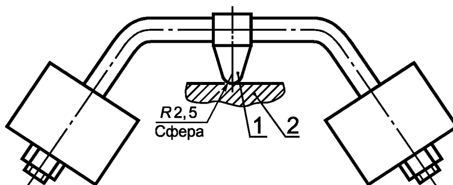
Рисунок 6 — Устройство для вдавливания шарика
