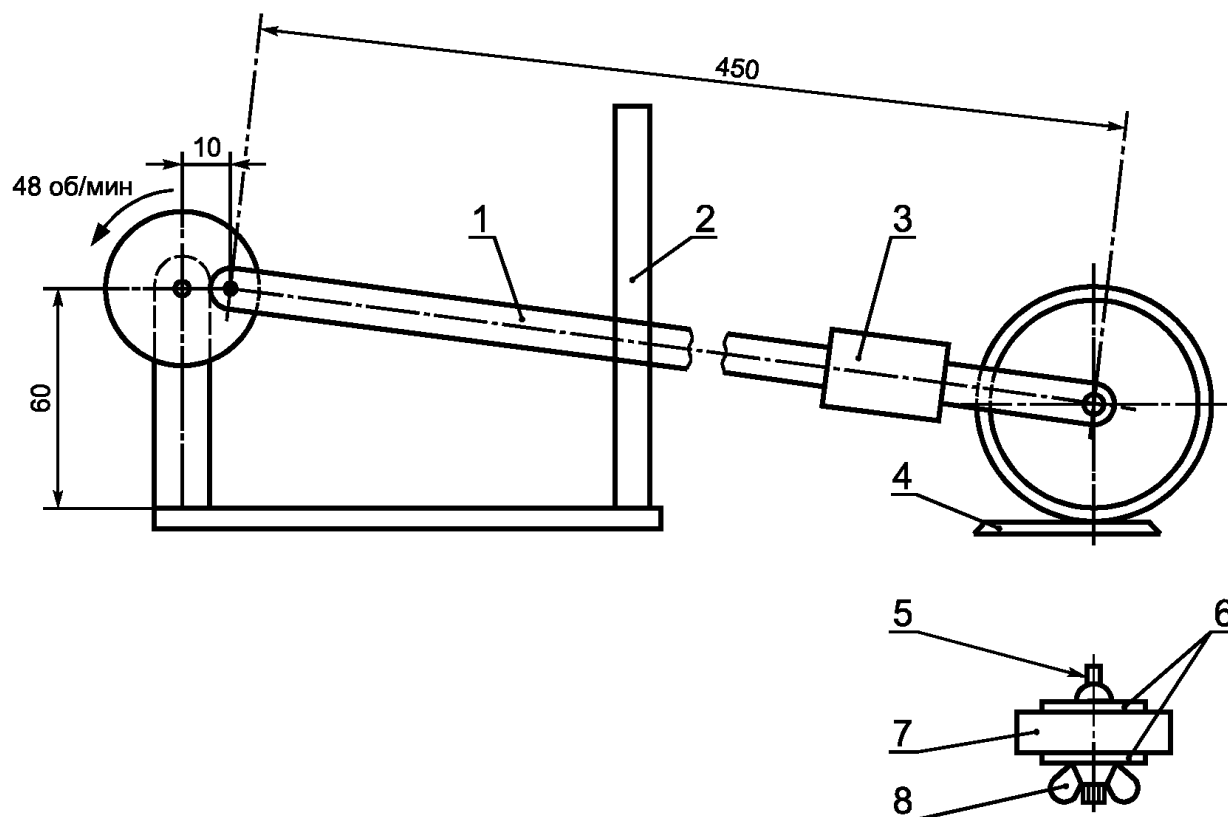
Рисунок 7 — Схема устройства для испытания горением
