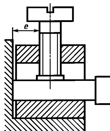
Зажим с прижимной пластиной
