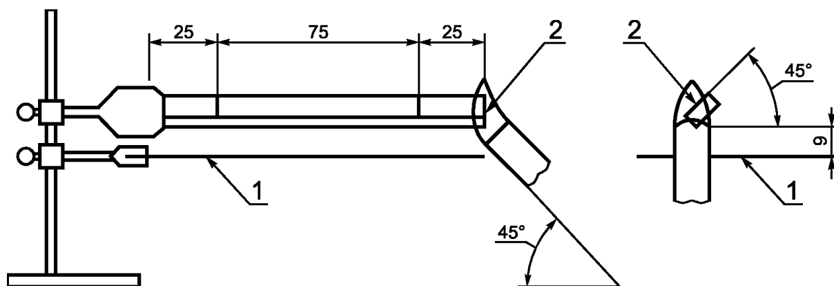
Рисунок 6 — Устройство для вдавливания шарика
