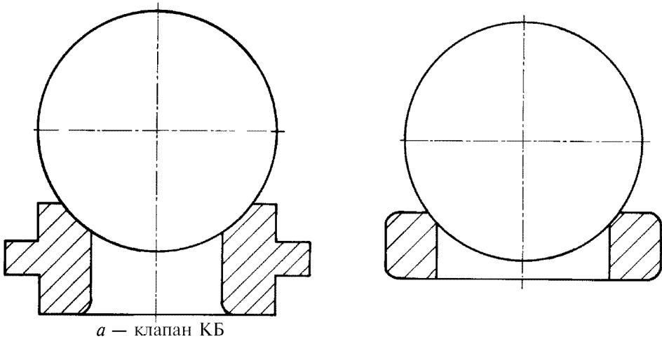
Рисунок 16 — Конструктивное исполнение седел клапанов
