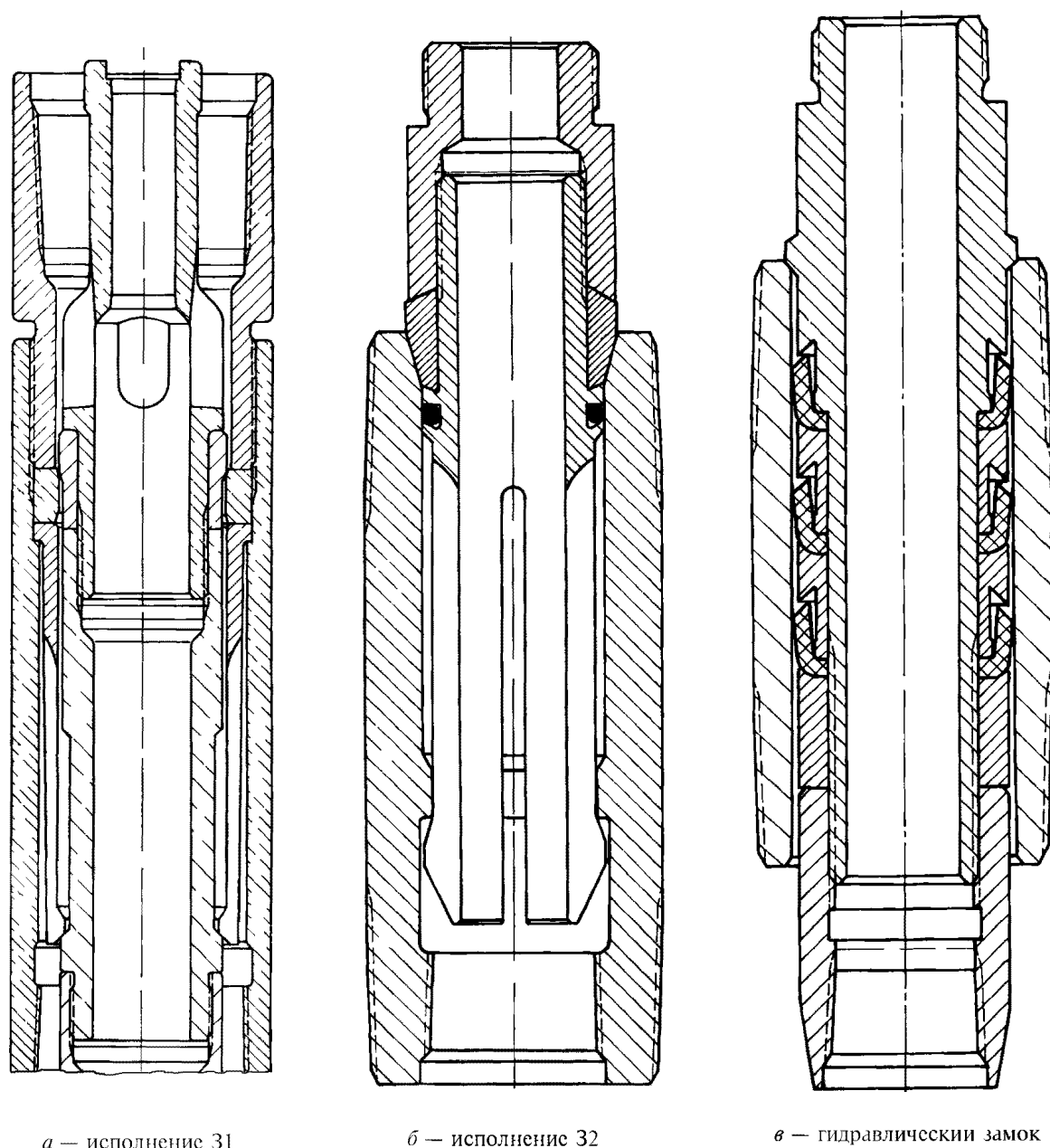
Рисунок 17 — Замки
