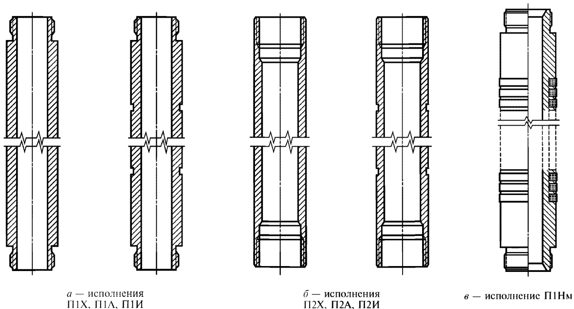
Рисунок 15 — Плунжеры
