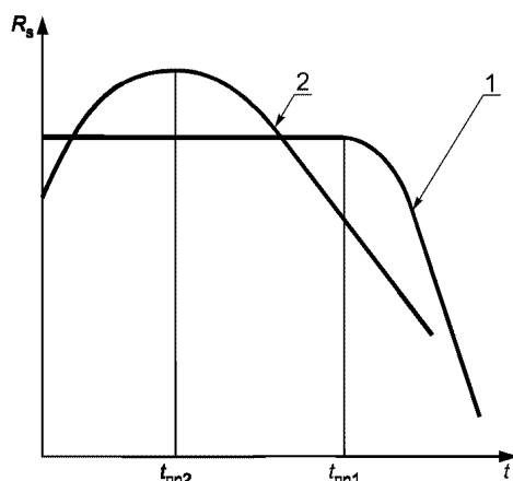
Рисунок В.2 — Определение времени проникания t_{\text{пр}} агрессивных сред по различным видам записываемых потенциометром кривых изменения во времени поверхностного электрического сопротивления R_s
