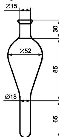
Рисунок 2 — Колба специальная для титрования
