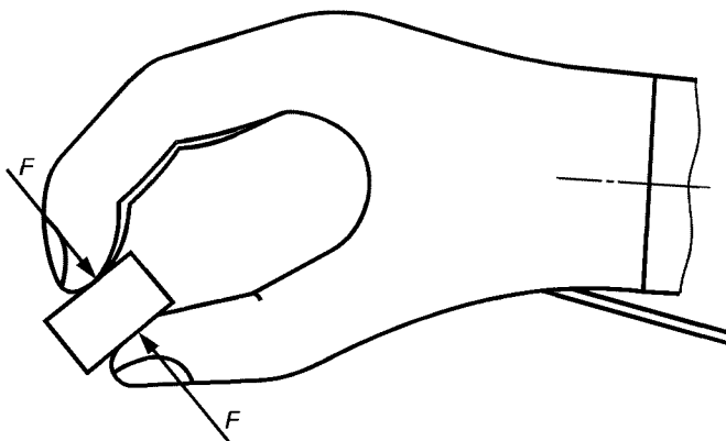
Рисунок 11 — Измерение усилия схвата
