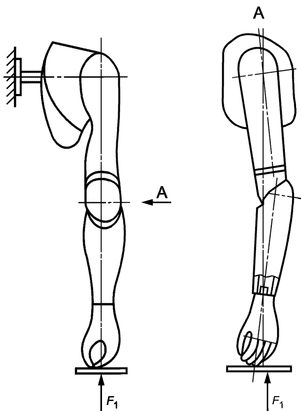
Рисунок 5 — Схема испытания на осевое нагружение концевого устройства
