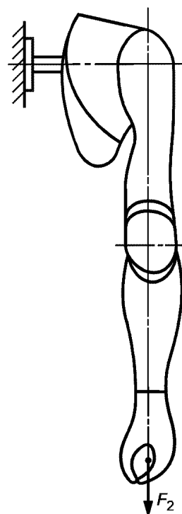
Рисунок 6 — Схема испытания на растяжение
