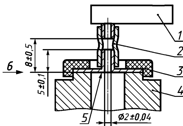
1 — слуховой аппарат (модульной конструкции); 2 — соединительная трубка; 3 — фиксатор; 4 — имитатор закрытого уха; 5 — наконечник; 6 — опорная плоскость имитатора закрытого уха
