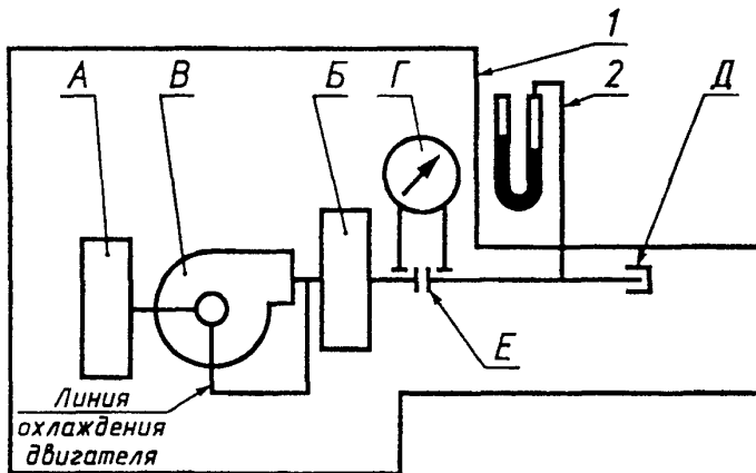
СХЕМА ИСПЫТАНИЯ УСТАНОВОК ФВУ А (наружное размещение)
