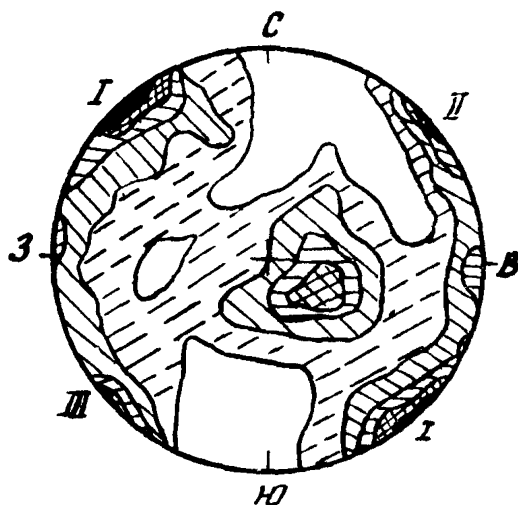
Рис. 4. Диаграмма трещиноватости в изолиниях: I-III - системы трещин (I - вертикальные, \beta СВ 50^\circ ; II - вертикальные, \beta ЮВ 130^\circ ; III - наклонные, \beta СВ 25^\circ , азимуты падения ЮВ \alpha 20^\circ . Количество точек от общего числа измерений (%): - (6-5); - (5-4), - (4-3), - (3-2), - (2-1), - (1-0)
