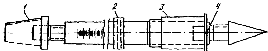
Рис. 1. Пенетромметр для испытания грунтов в скважинах (конструктор Б.А.Биневич):
