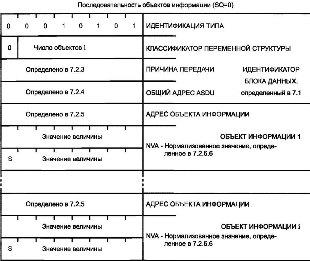
Рисунок 36 — ASDU. M_ME_ND_1. Значение измеряемой величины, нормализованное значение без описателя качества
