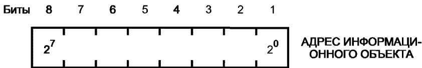
Рисунок 9 — АДРЕС ИНФОРМАЦИОННОГО ОБЪЕКТА (один байт)
