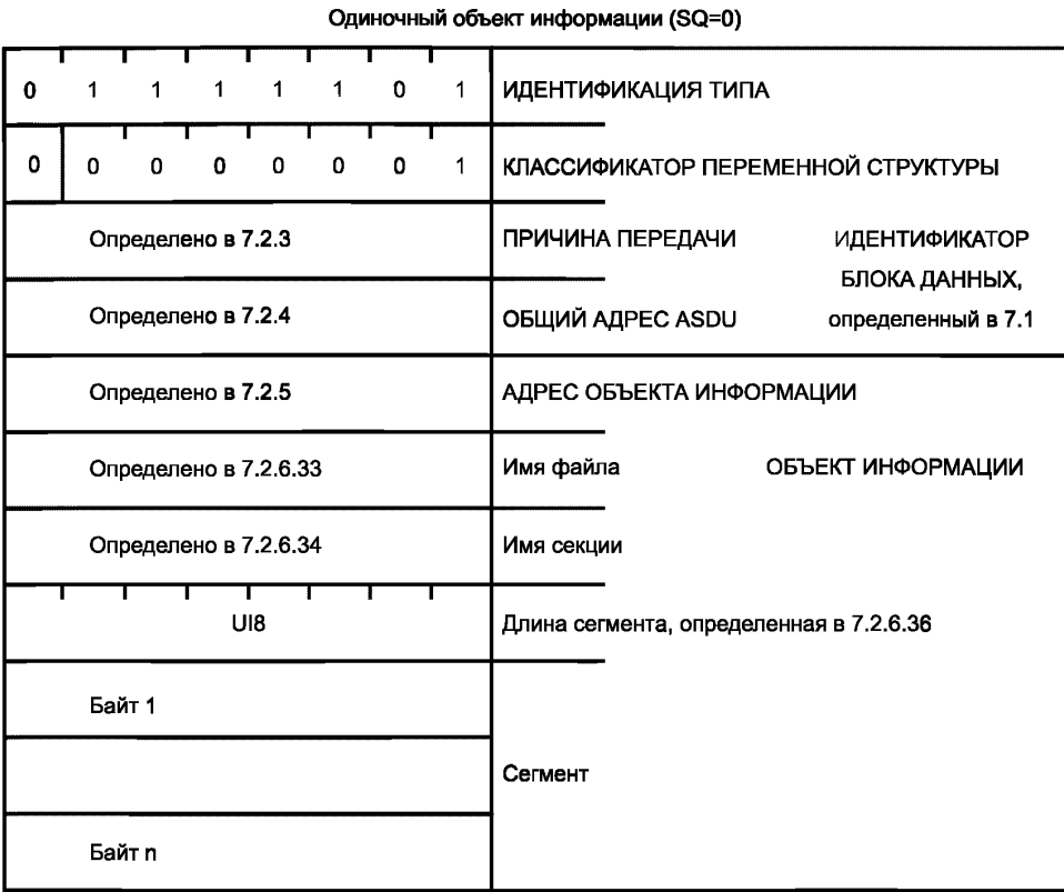
Рисунок 62 — ASDU. F_SG_NA_1. Сегмент
