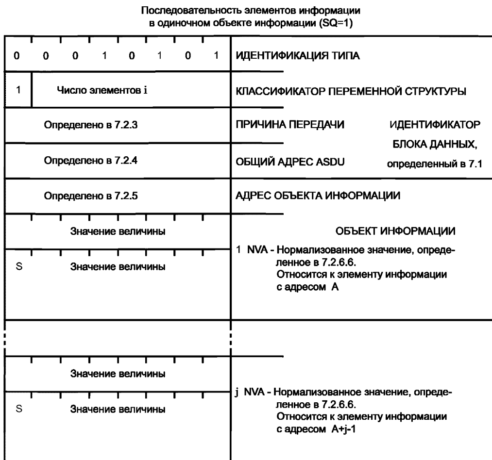
Рисунок 37 — ASDU. M_ME_ND_1. Последовательность значений измеряемых величин, нормализованных величин без описателя качества
