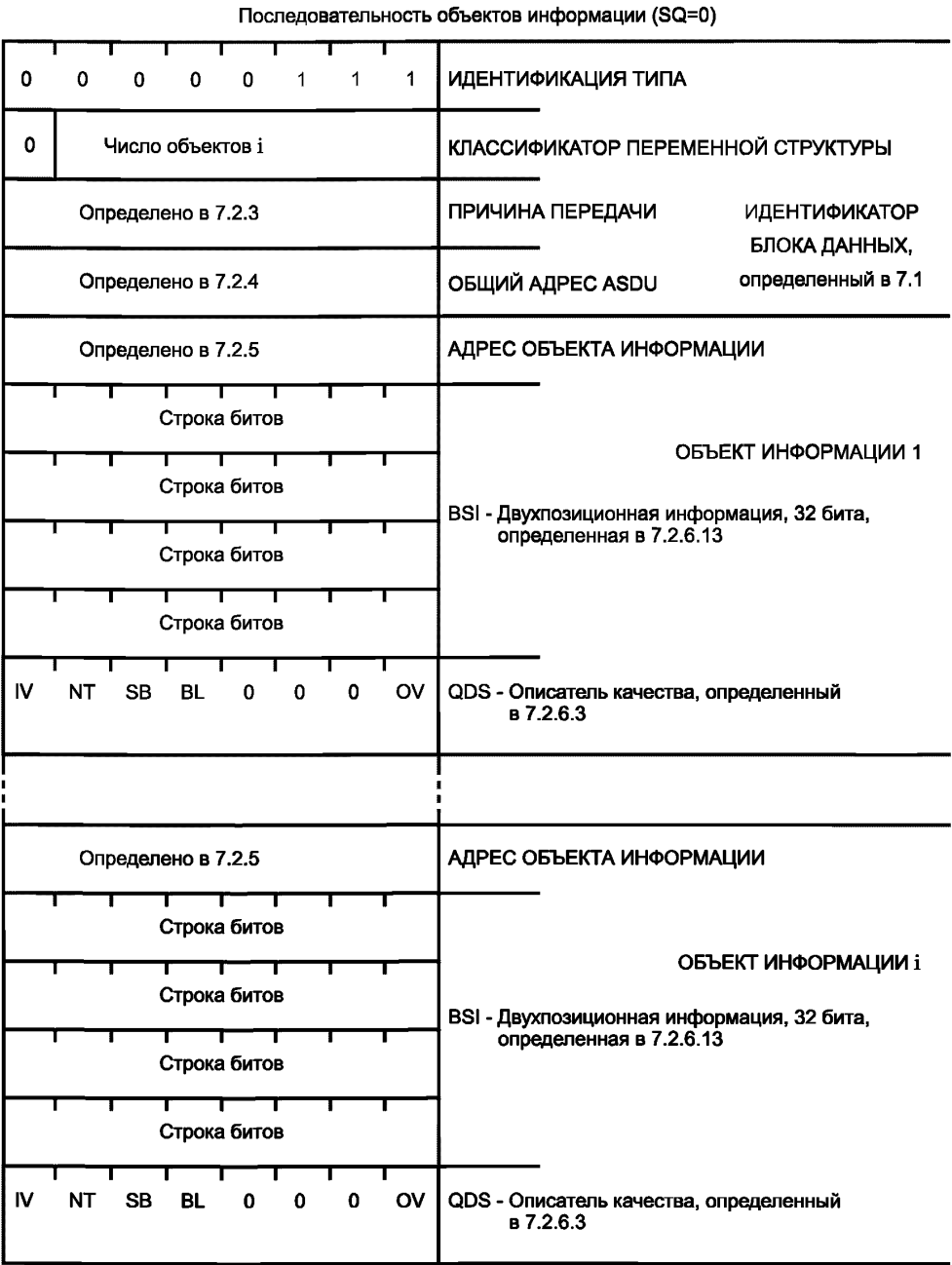
Рисунок 20 — ASDU. M_BO_NA_1. Строка из 32 битов
