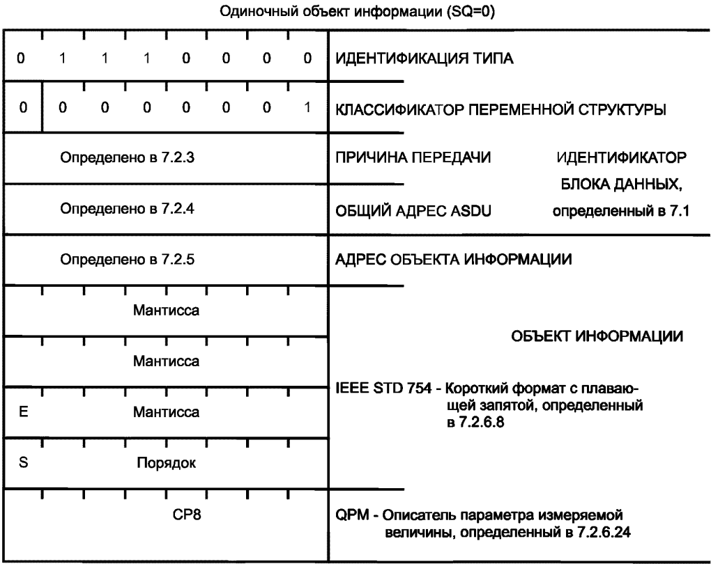
Рисунок 55 — ASDU. P_ME_NC_1. Параметры измеряемых величин, короткий формат с плавающей запятой
