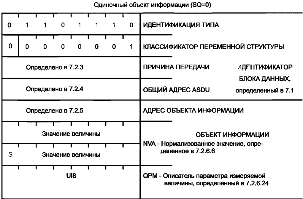
Рисунок 53 — ASDU. P_ME_NA_1. Параметры измеряемых величин, нормализованное значение
