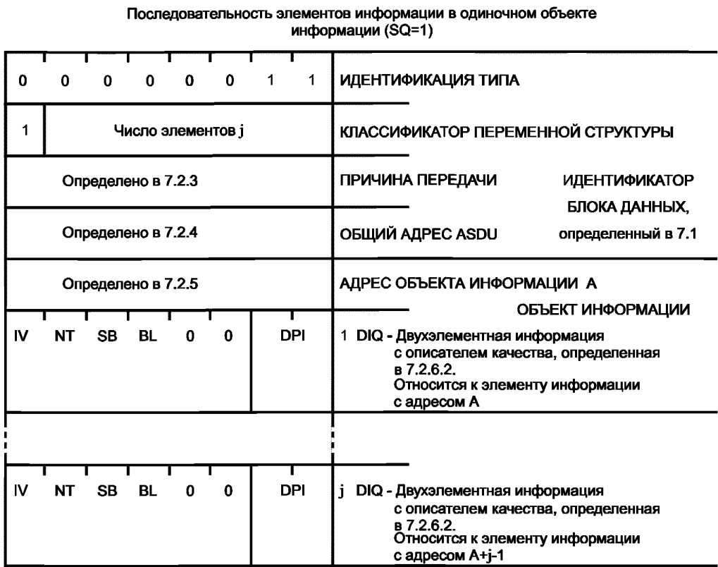
Рисунок 16 — ASDU: M_DP_NA_1. Последовательность двухэлементной информации без метки времени
