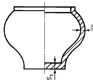
Рисунок 2 — Горшок
