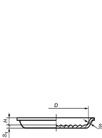
Рисунок 7 — Сковорода-гриль
