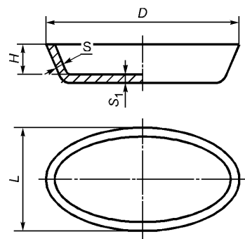
Рисунок 9 — Рыбница
