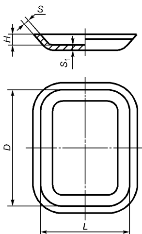
Рисунок 8 — Противень
