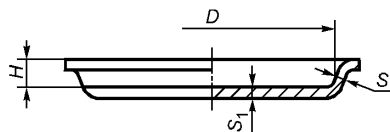
Рисунок 5 — Сковорода
