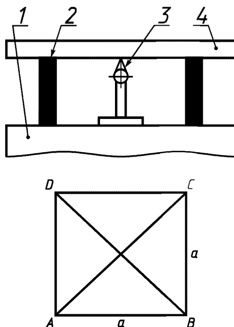
1 — плита; 2 — равновысокие опоры; 3 — индикатор; 4 — поверочная линейка
