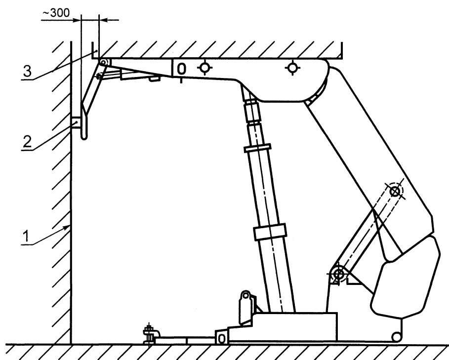
Рисунок А.9 — Схема нагружения оградительного щита
