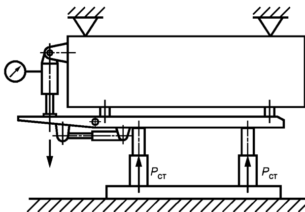
Рисунок А.2 — Схема нагружения гидроподжимного козырька перекрытия
