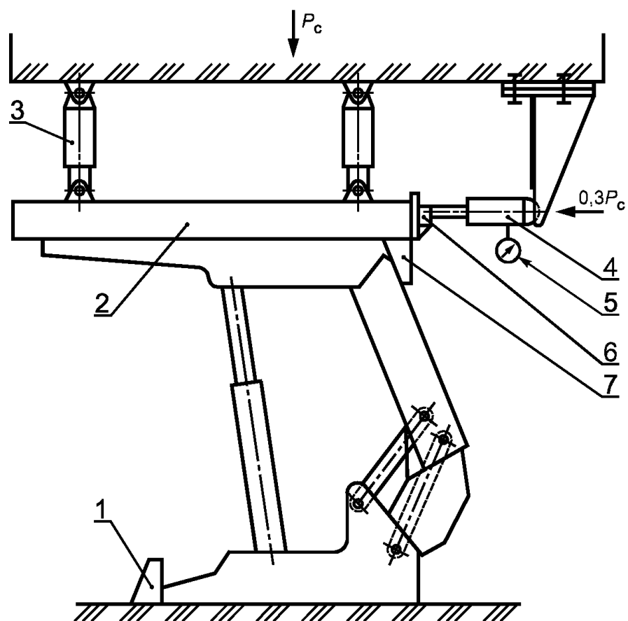
1 — упор; 2 — рама; 3, 4 — гидродомкраты; 5 — манометр; 6 — тензоопора; 7 — упор
