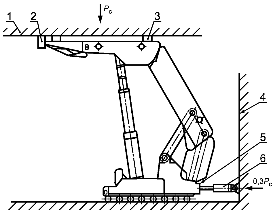
1 — нагрузочная плита; 2 — упор; 3, 5 — тензоопоры; 4 — колонна стенда; 6 — гидродомкрат
