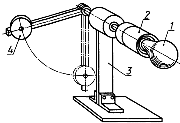
1 — лампа; 2 — патрон; 3 — стойка; 4 — противовес
