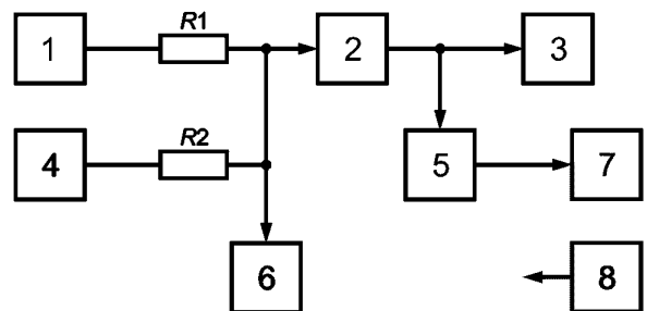
1 — генератор сигналов НЧ; 2 — передатчик; 3 — эквивалент антенны; 4 — генератор сигналов НЧ; 5 — элемент связи; 6 — милливольтметр НЧ; 7 — модулометр; 8 — анализатор спектра ВЧ; R1, R2 — резисторы сопротивлением (6,8 \pm 0,34) кОм
