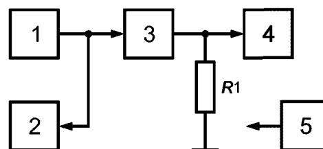
1 — генератор сигналов НЧ; 2 — милливольтметр НЧ; 3 — возбудитель передатчика; 4 — милливольтметр ВЧ; 5 — анализатор спектра ВЧ; R1 — резистор сопротивлением (75±4) Ом
