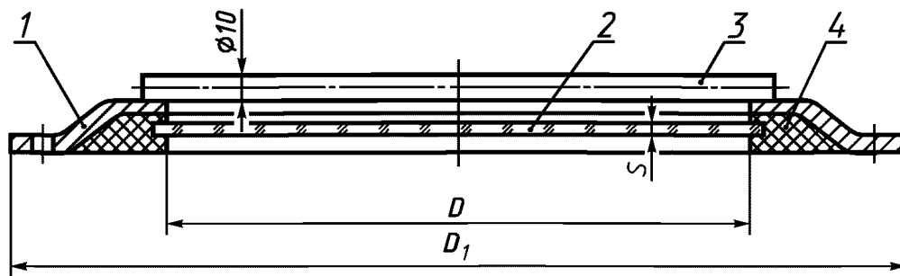
1 — корпус; 2 — стекло; 3 — прутки; 4 — герметизирующий материал
