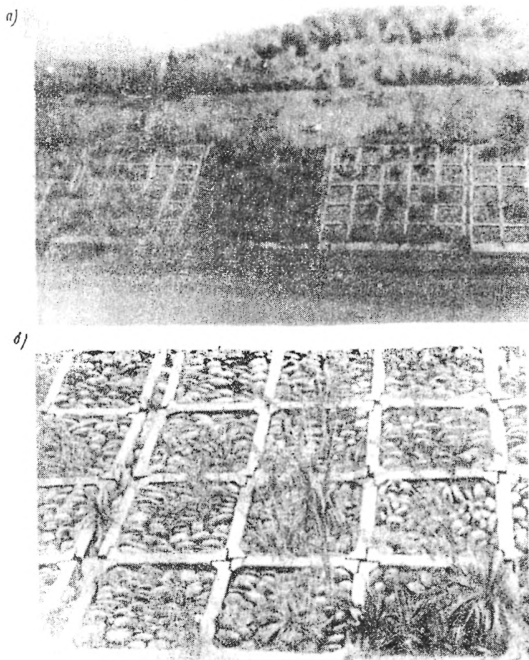
Рис.1. Укрепление откосов выемки решетчатыми конструкциями - ми на автомобильной дороге в районе Северного Кавказа : а-общий вид; б-секция с ячейками, заполненными местным кам- нем
