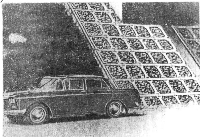
Рис.8. Укрепление конусов путепроводов на автомобильной дороге;
