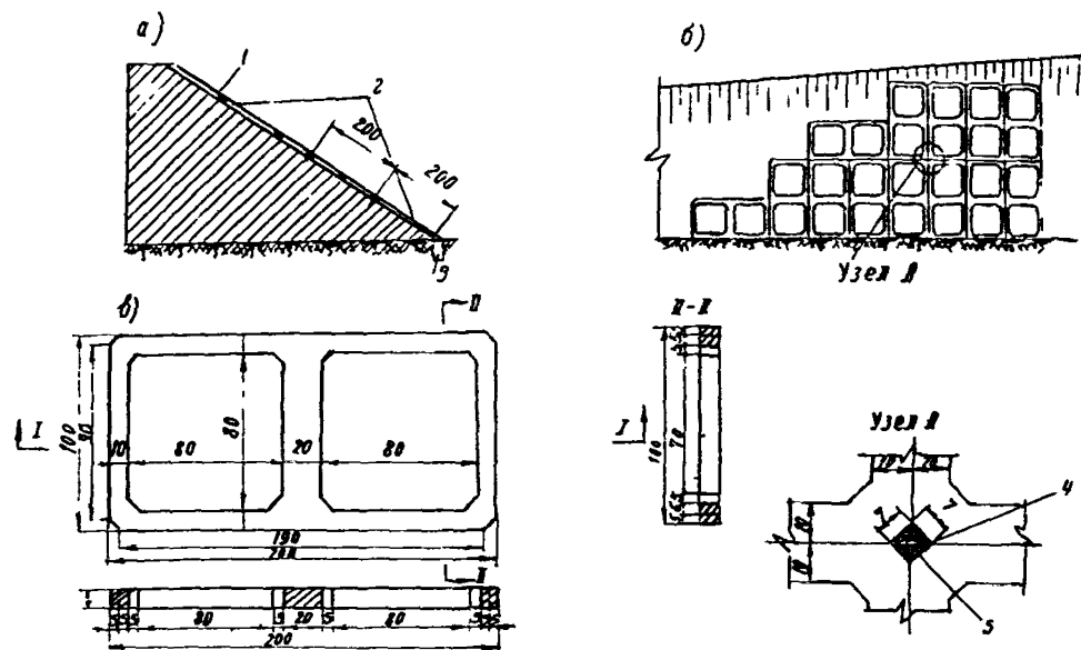
Рис.7. Укрепление откосов железобетонной рамой (вариант №8): а-поперечный разрез; б-план; в-железобетонная рама; 1-заполнение ячеек (засев трав); 2-железобетонные решетки; 3-бетонный упор (при мокрых и подтопляемых откосах); 4-омо- ноличивание цементным раствором; 5-металлический штырь.
