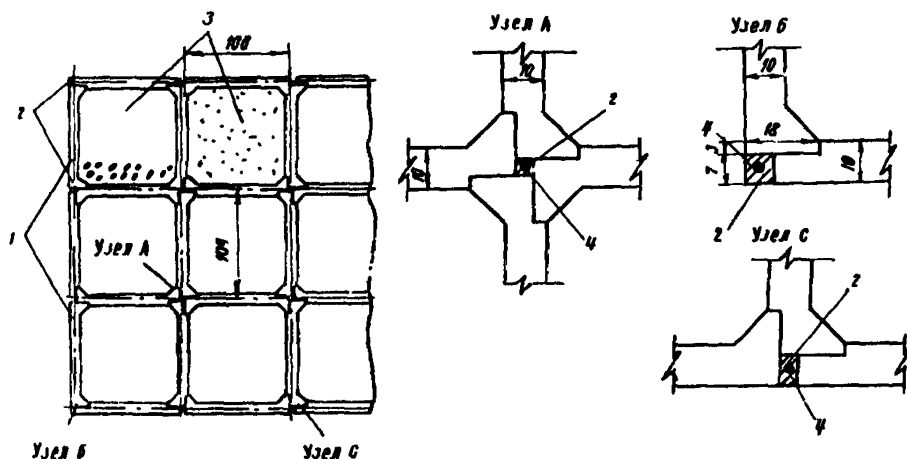
Рис.5. Решетчатая конструкция с прямоугольным расположением элементов (вариант № 2): 1-сборный элемент; 2-омоноличивание цементным раствором ; 3-заполнение ячеек (каменная наброска, посев трав и т.д.); 4-металлическая свая
