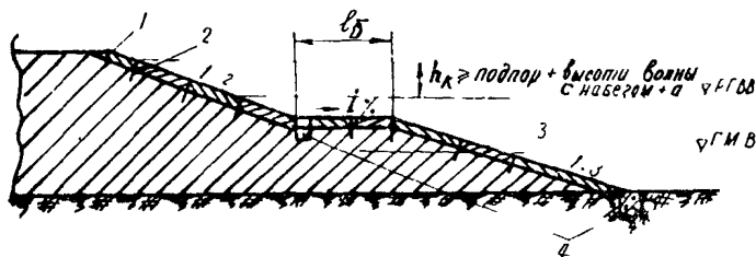
Рис.4. Схема укрепления пойменных насыпей высотой более 8м сборными решетчатыми конструкциями:
