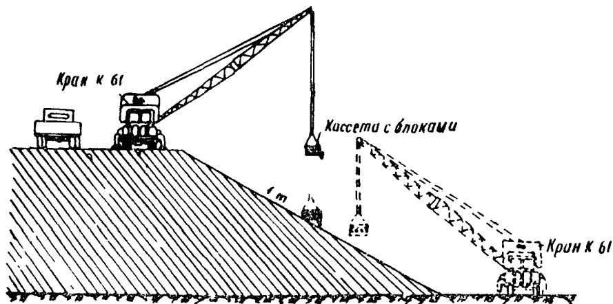
Рис.5. Схема укладки сборных элементов на поверхность откосов краном К-61
