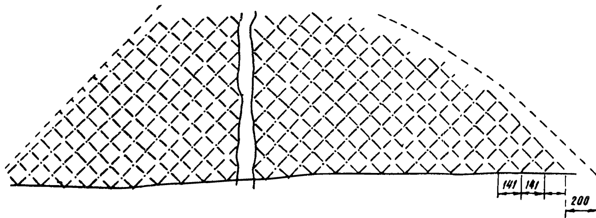
Рис.12. Разбивка откоса выемки под укладку сборных элементов
