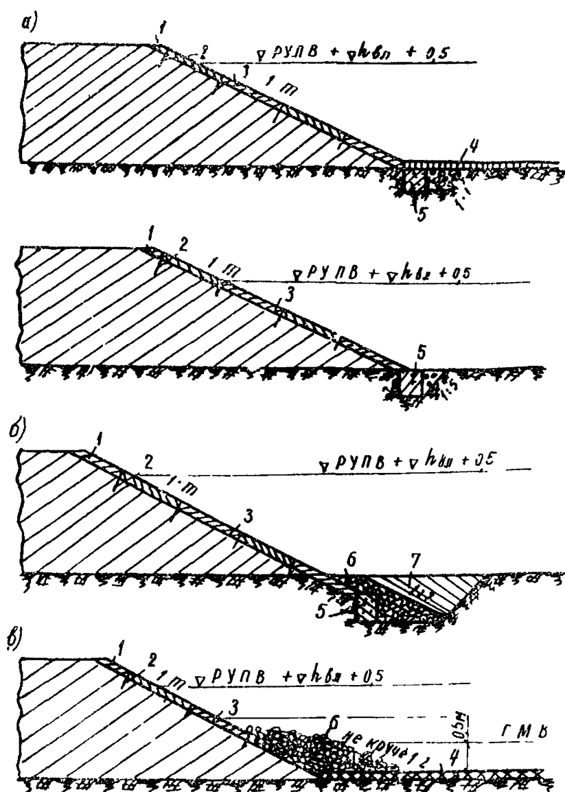
Рис.3. Схемы укрепления откосов пойменных насыпей решетчатыми конструкциями: а- при отсутствии размывов у подошвы пойменных насыпей и отсутствии меженных вод; б-при размывах у подошвы насыпей и отсутствии меженных вод; в- при отсутствии размыва у подошвы насыпей и при наличии меженных вод; 1-засев трав с плакировкой; 2-сваи металлические; 3-бетонная решетка; 4-гибкое укрепление; 5-бетонный упор 0,3х0,4м; 6-каменная наброска; 7-обратная засыпка
