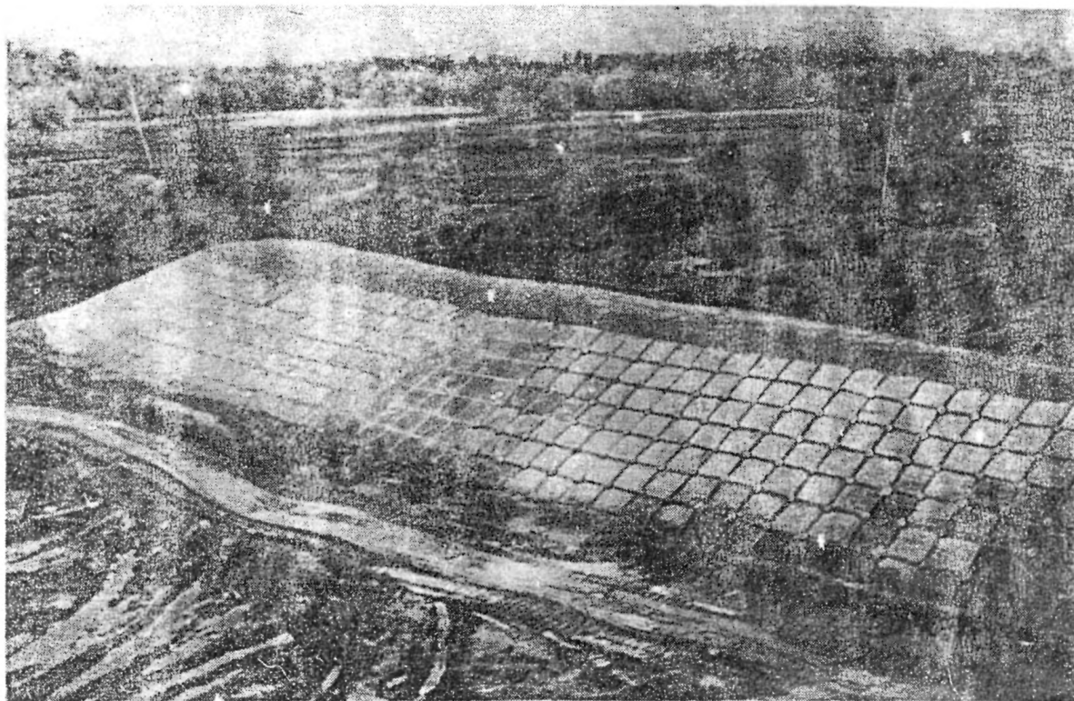
Рис.2. Укрепление откосов дамбы решетчатыми конструкциями с заполнением ячеек цементогрунтом и нефтегрунтом на автомобильной дороге в Тюменской области
