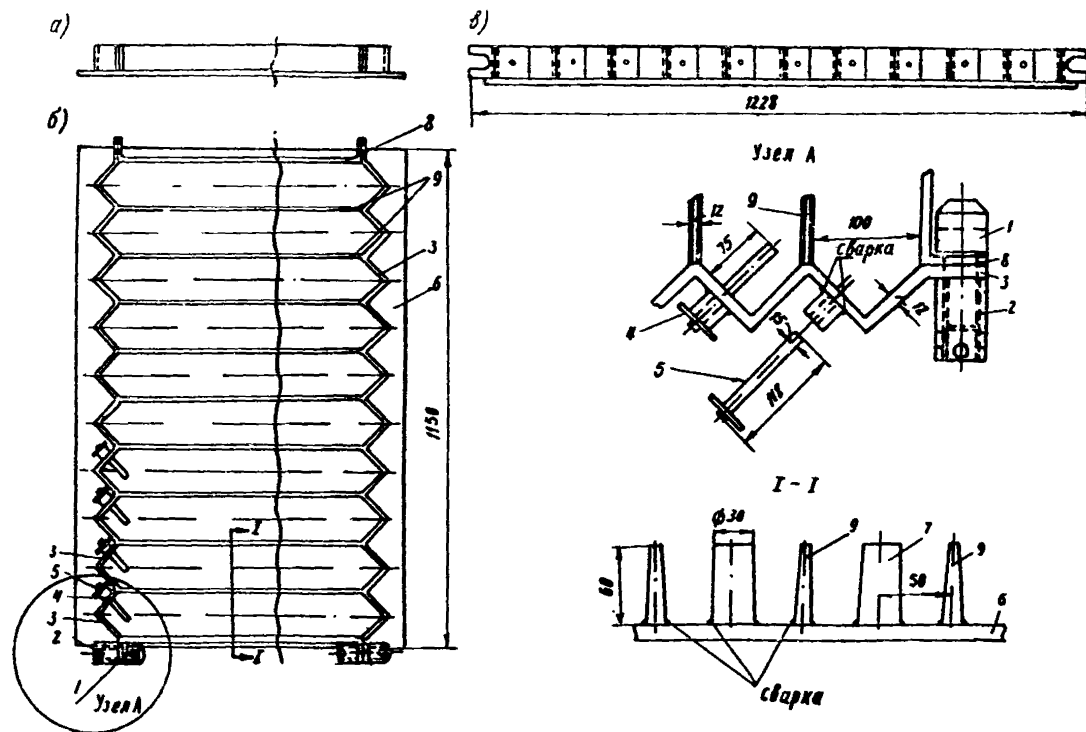
Рис.10. Металлическая опалубка для сборных элементов:
