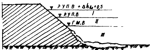
Рис.2. Схема определения зон укрепления откосов подтопляемых насыпей : I-зона паводкового волнового воздействия; II-зона паводкового подтопления; III-зона постоянного уровня подтопления;
