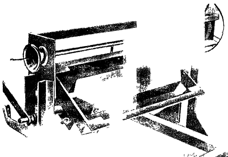
Рис.11. Вибромашина Купавинского завода ЖБК треста "Центр-дорстрой"
