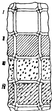
Рис.1. Рекомендуемые типы заполнения ячеек решетчатых конструкций : I-растительный грунт с засевом трав ( h = 10\text{см} ); II-грунт, обработанный 8% битума ( h = 10\text{см} ); III-каменная наброска (размером 70-200мм); IV-моноплитный бетон марки "200" ( h = 10\text{см} ) на песчаной или щебеночной подготовке ( h = 10\text{см} )
