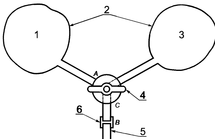
1 — ПГС; 2 — газовые емкости; 3 — чистый воздух; 4 — двухходовой кран; 5 — газовый вход прибора или пробоотборный зонд; 6 — соединение с прибором
