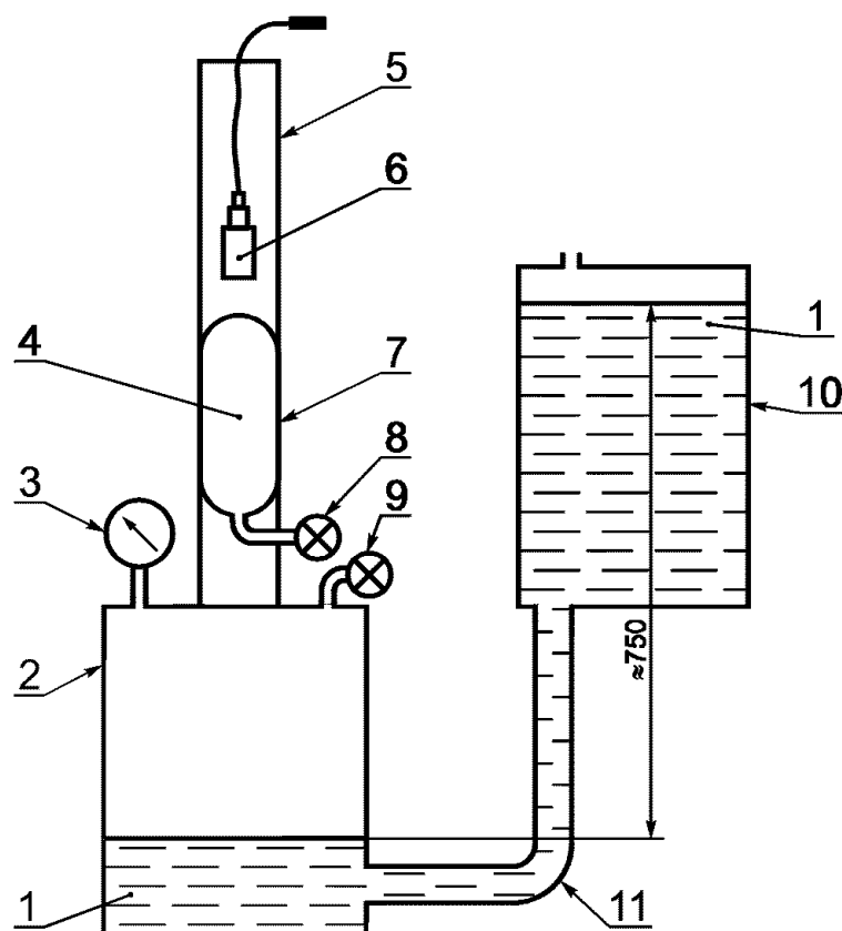
Рисунок В.6 — Схема установки, обеспечивающей скачкообразный переход из чистого воздуха в газозоудную смесь
