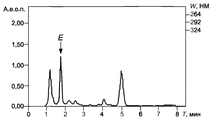
Рисунок А.3 — Хроматограмма экстракта витамина Е
