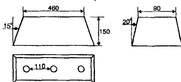
Рис.3. Эскиз отражателя для ОСП.
