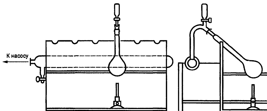
Рисунок 1 — Аппарат для мокрого окисления пробы
