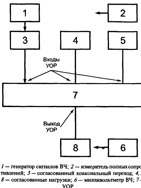
Рисунок 2 — Схема определения КПД
