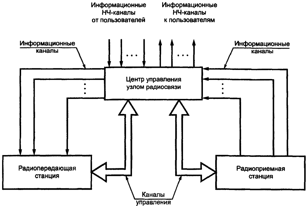
Рисунок А.1 — Упрощенная структурная схема УРС
