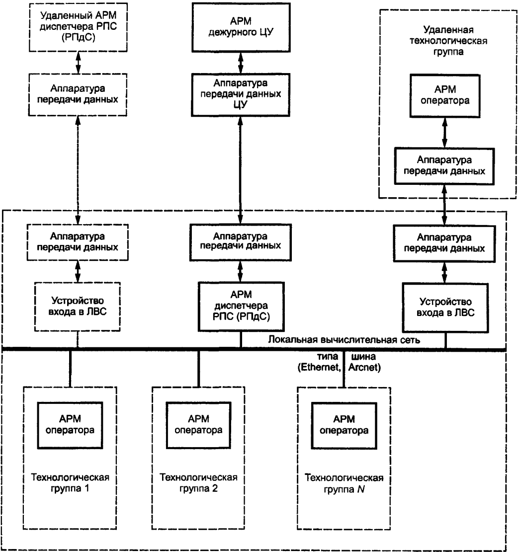
Рисунок 3 — Структурная схема системы управления на уровне РПдС (РПС) для ЛВС типа шина
