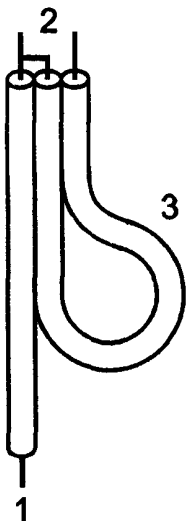
1 — несимметричный вход; 2 — симметричный выход; 3 — полуволновая петля
