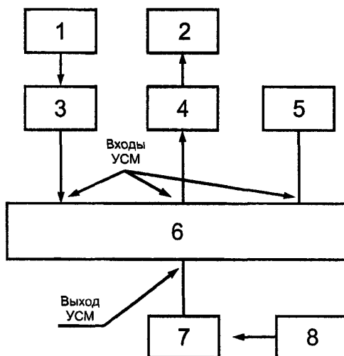
Рисунок 1 — Схема определения развязки между входами УСМ
