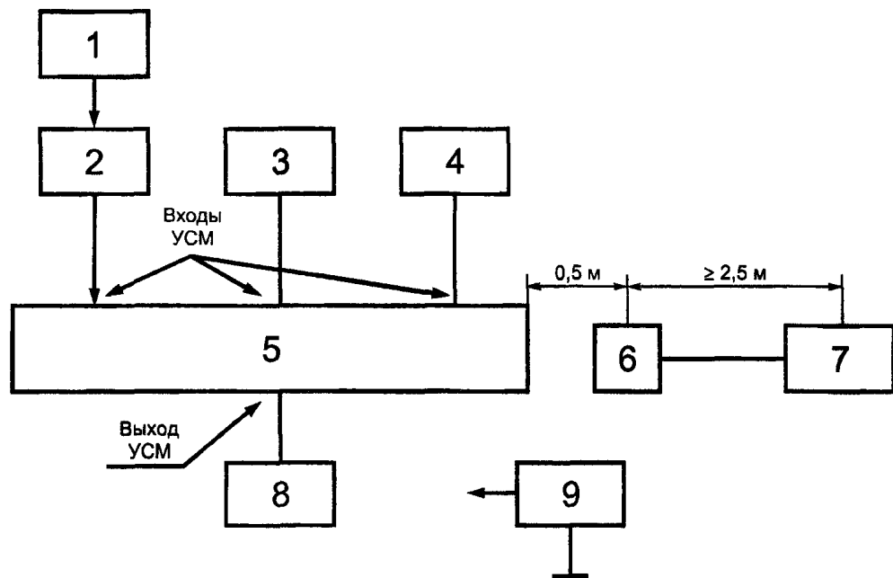
1 — генератор сигналов ВЧ; 2 — согласованный коаксиальный переход; 3, 4, 8 — экранированные согласованные нагрузки; 5 — УСМ; 6 — измерительная антенна; 7 — измеритель напряженности ЭМП; 9 — милливольтметр ВЧ
