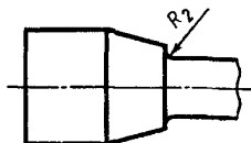
Рисунок 2 — Головка образца с переходным участком
