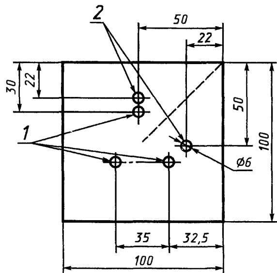
1 — опорные штифты; 2 — установочные штифты
