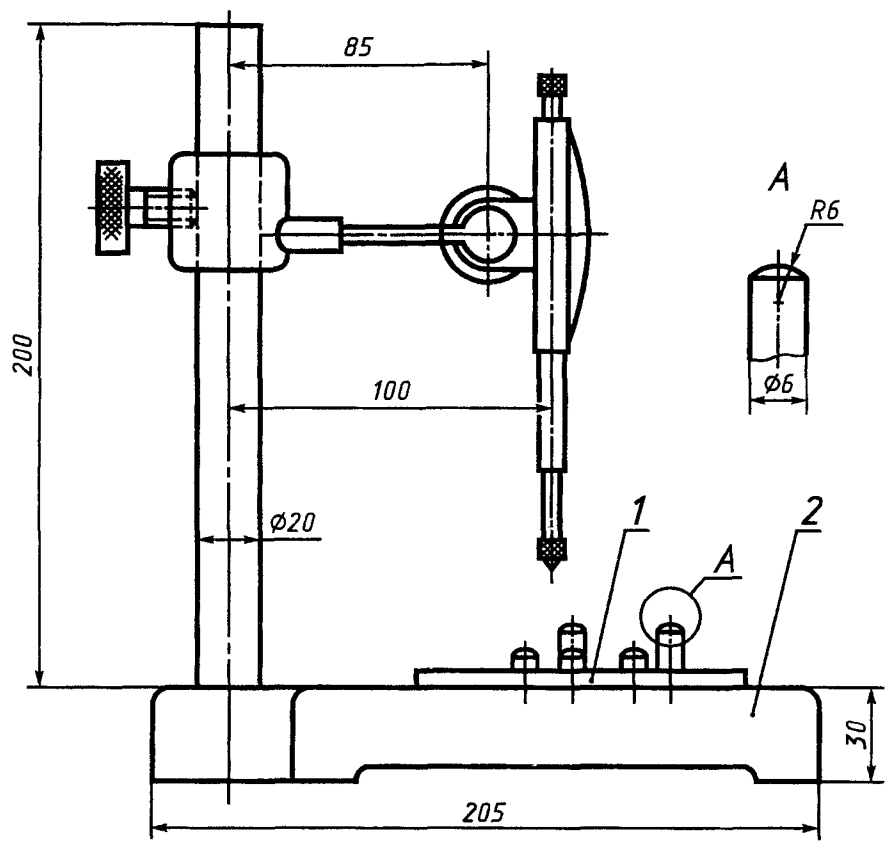
1 — подставка; 2 — опорная плита
