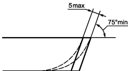
Рисунок 2 — Угол схождения обуха и лезвия клинка
