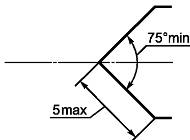
Рисунок 1 — Угол схождения боковых граней острия клинка
