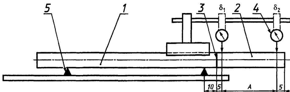
Рисунок 4 — Схема измерения отклонения от соосности трубы и приварных концов
