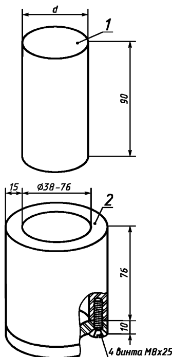
1 — пуансон; 2 — форма
