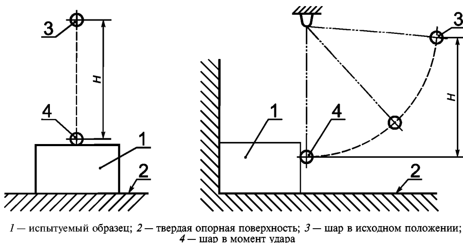
Рисунок 1 — Испытания на удар с помощью стального шара
