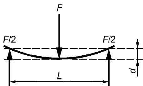
L — испытуемая длина, расстояние между двумя опорами; F — сила изгиба (реакция силы изгиба), приложенная под прямым углом к испытуемому образцу; d — изгиб (стрела прогиба) посередине между движущимися опорами
