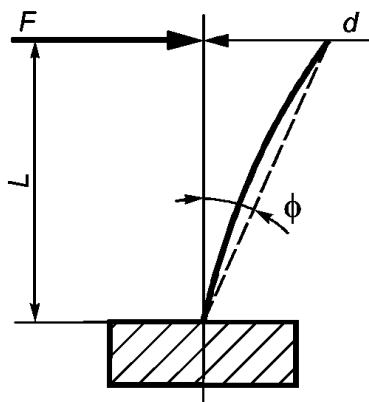
L — испытуемая длина (длина изгиба), расстояние между верхней линией зажима и изгибающим зондом; F — сила изгиба (реакция силы изгиба), приложенная к испытуемому образцу с помощью подвижного зонда; d — изгиб (стрела прогиба) или длина перемещения подвижного зонда; \phi — арктангенс d/L — угол отклонения
