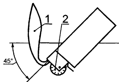
1 — пламя; 2 — искрообразующее колесико
