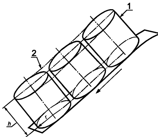
Рисунок 9 — Определение зоны безопасности горки
