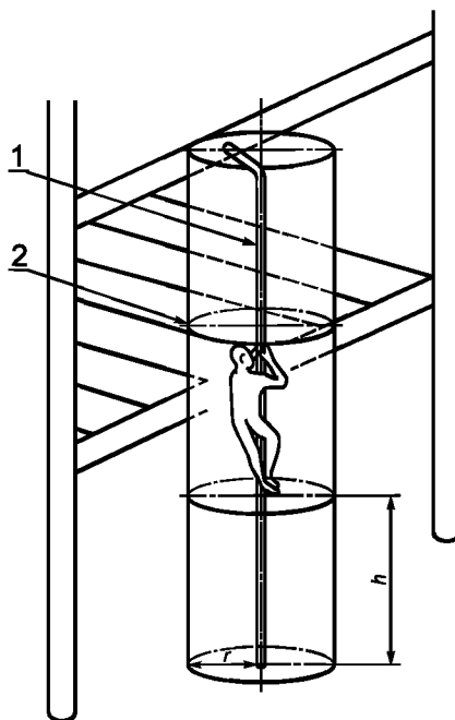
Рисунок 10 — Определение зоны безопасности шеста
