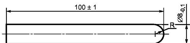
Рисунок Г.12 — Стержень-палец А (малый)
