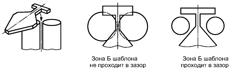
Рисунок Г.6 — Испытания прямоугольных зазоров с использованием зоны Б шаблона
