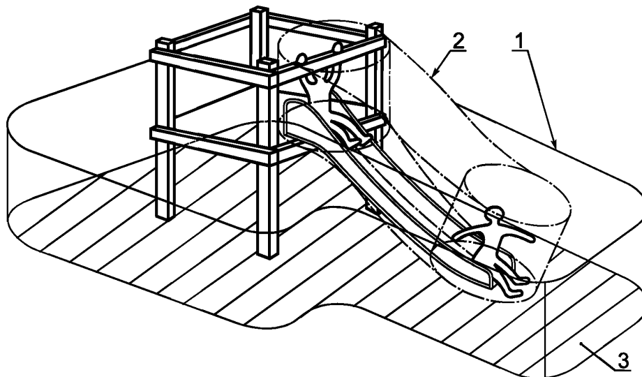
1 — игровая зона; 2 — зона безопасности; 3 — зона приземления
