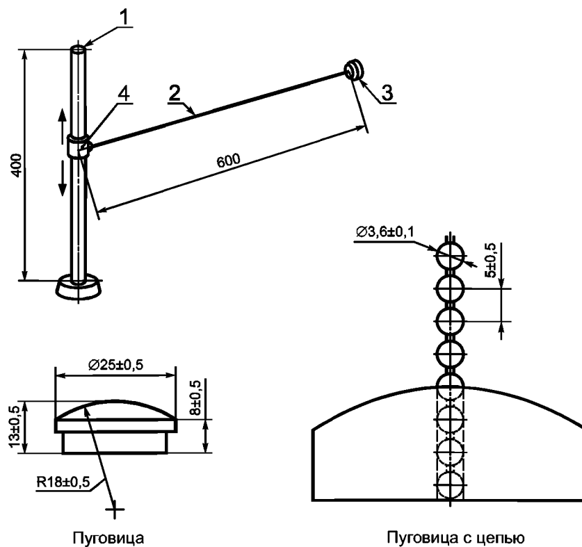
Рисунок Г.9 — Испытательное устройство для испытаний застревания пуговицы
