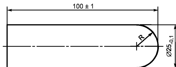
Рисунок Г.13 — Стержень-палец Б (большой)
