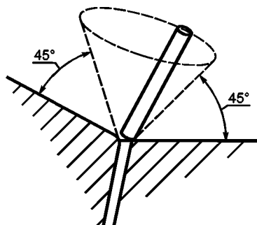
Рисунок Г.14 — Схема вращения стержня-пальца
