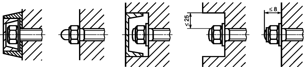
Рисунок 4 — Защита болтовых соединений
