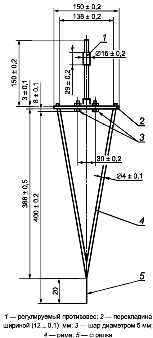
Рисунок 1 — Маятник Кенига
