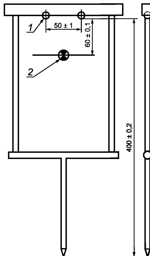
Рисунок 2 — Маятник Персоза
