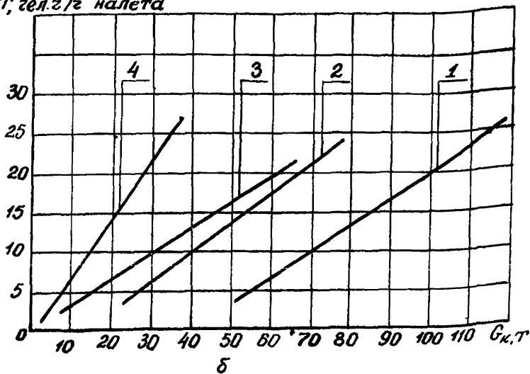
Рис. 3. Удельная трудоемкость технического обслуживания ВС в зависимости от массы конструкции вертолетов I-III классов (а) и самолетов I-IV групп (б); I-3 - класс вертолета; I-4 - группа самолета
