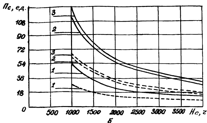
Рис. 6. Пропускная способность одного ангарного места стоянки воздушных судов, находящихся в эксплуатации, Ми-8 (1), Як-40 (2) и Л-410 (3): а - в АТБ, имеющей не более двух типов ВС в приписном парке; б - в АТБ с многотипным приписным парком
