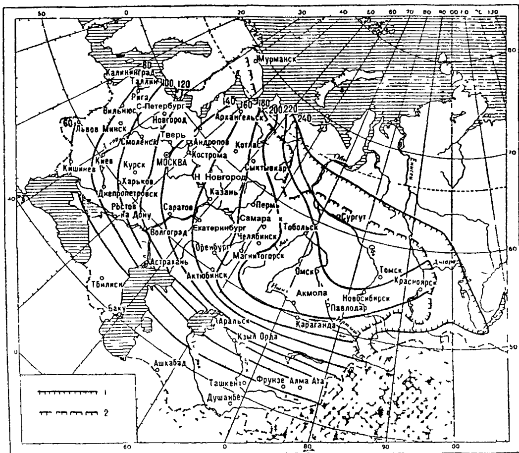
Рис 3.1 Карта изолиний глубины промерзания Z_{cp} грунтов, см 1 - граница сплошного распространения вечномёрзлых грунтов, 2 - то же островного (глубиной до 25 м) По состоянию на 1992г
