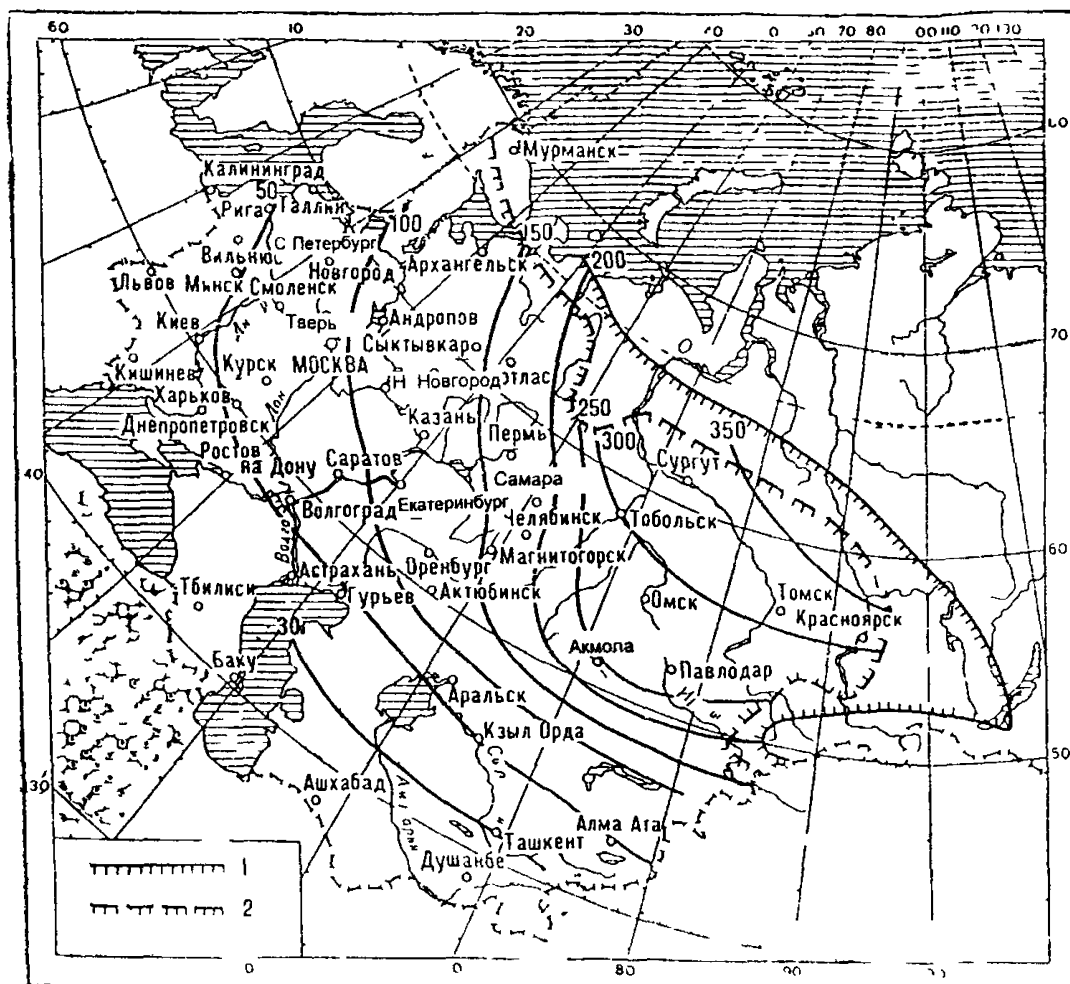
Рис 3 2 Карта изолиний климатического коэффициента \alpha_0 , см 2 /сут Поз 1 и 2 - см на рис 3 1 По состоянию на 1992г
