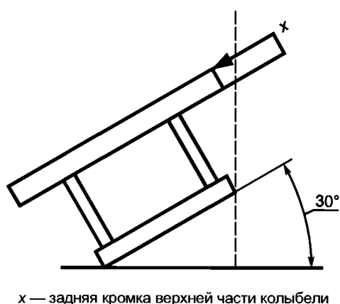
x — задняя кромка верхней части колыбели
