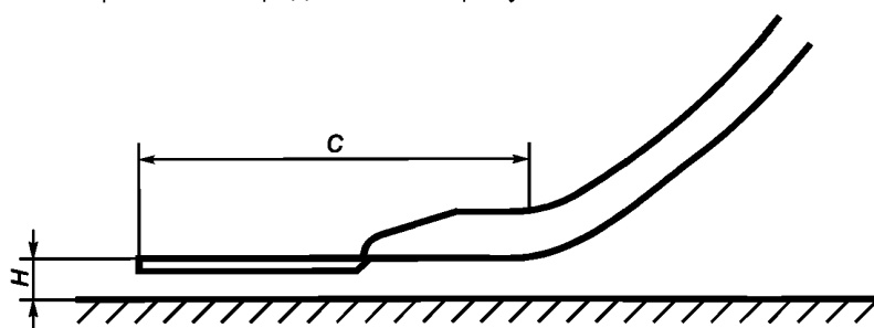
Рисунок 6 — Конечный участок горки типа 2
