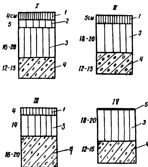
Рис.1. Типы конструкций дорожных одежд с основаниями из битумоминеральных смесей для дорог 1-IV категорий:
