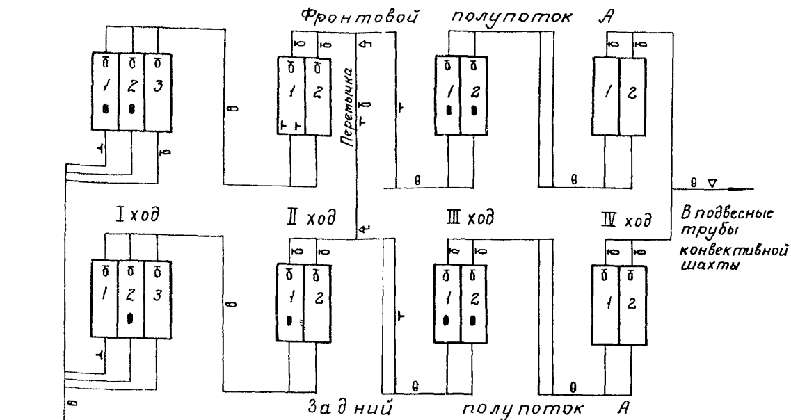
Рис. I. Схема экспериментального контроля НРЧ котла ТМР-314:
