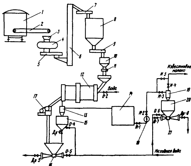
Рис.3-3. Схема разгрузки и хранения извести
