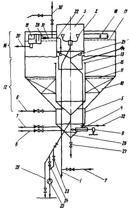
Рис.3-2. Устройство осветлителя ВТИ-1000 для известкования с коагуляцией, производительностью 100 м 3 /ч:
