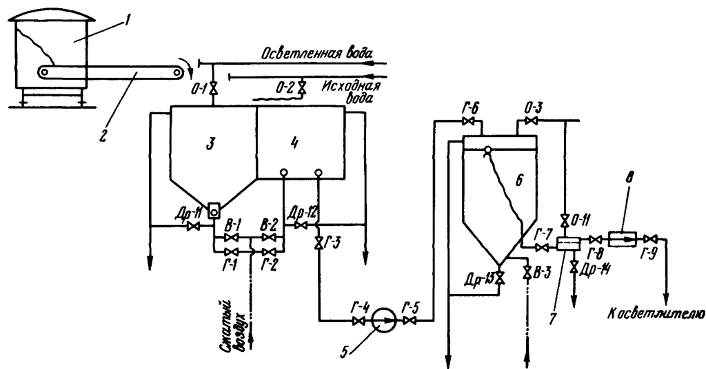
Рис.3-5. Схема приготовления и дозирования коагулянта (сернокислого железа)
