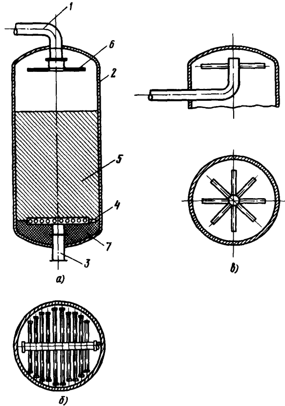
Рис.5-3. Устройство прямоточного монолитового фильтра:
