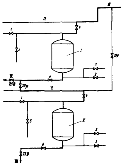
Рис.6-5. Схема последовательной регенерации фильтров:
