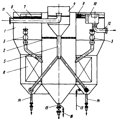
Рис.2-1. Схема осветлителя ЦНИИ-2 производительность 450 м 3 /ч
