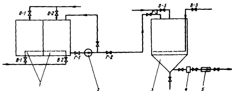
Рис.2-3. Схема приготовления и дозирования коагулянта - сернокислого алюминия
