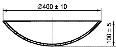
Рисунок 1 — Чаша для затворения
