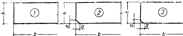
Рис. 2. Очертание ребер перемычек
