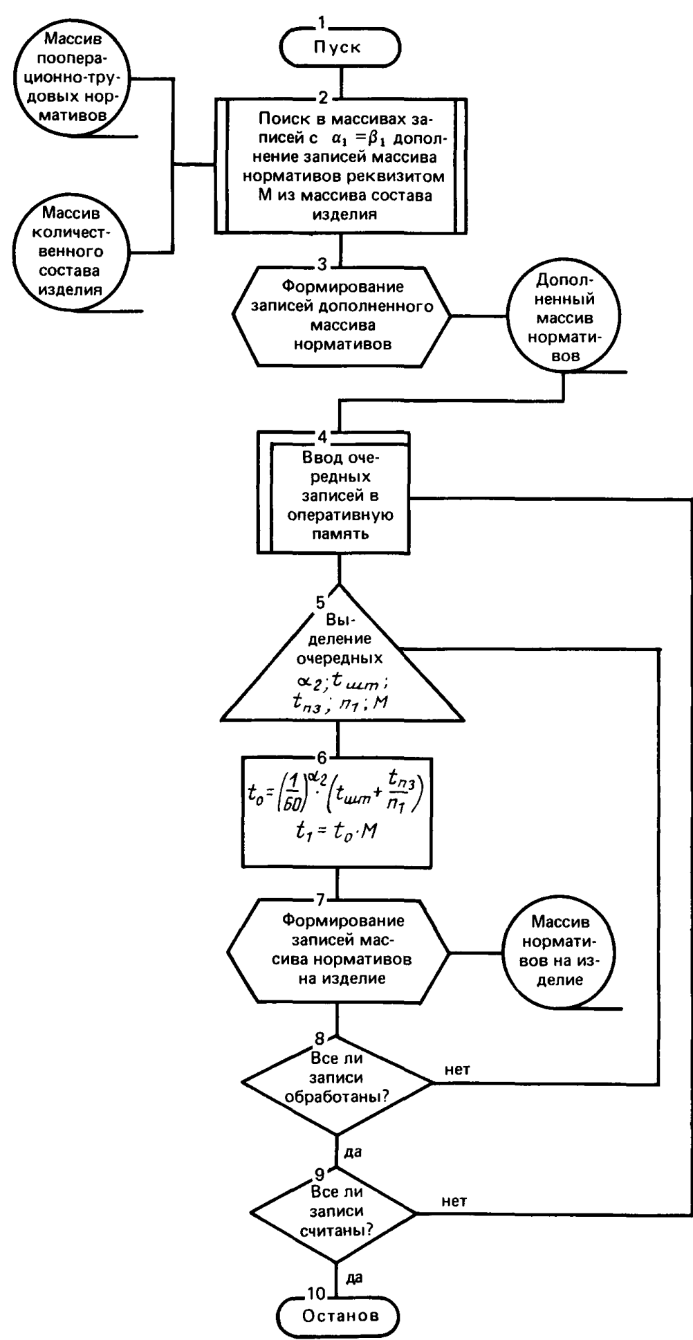
БЛОК-СХЕМА алгоритма создания пооперационного массива норм времени
