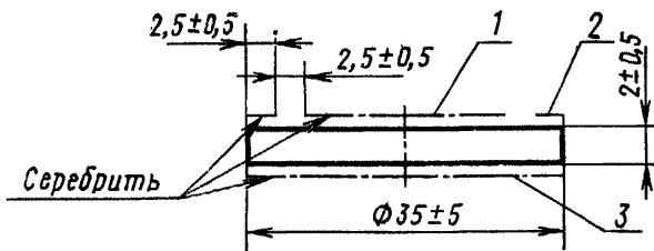
1—электрод низшего напряжения; 2—охранный электрод; 3— электрод высшего напряжения
