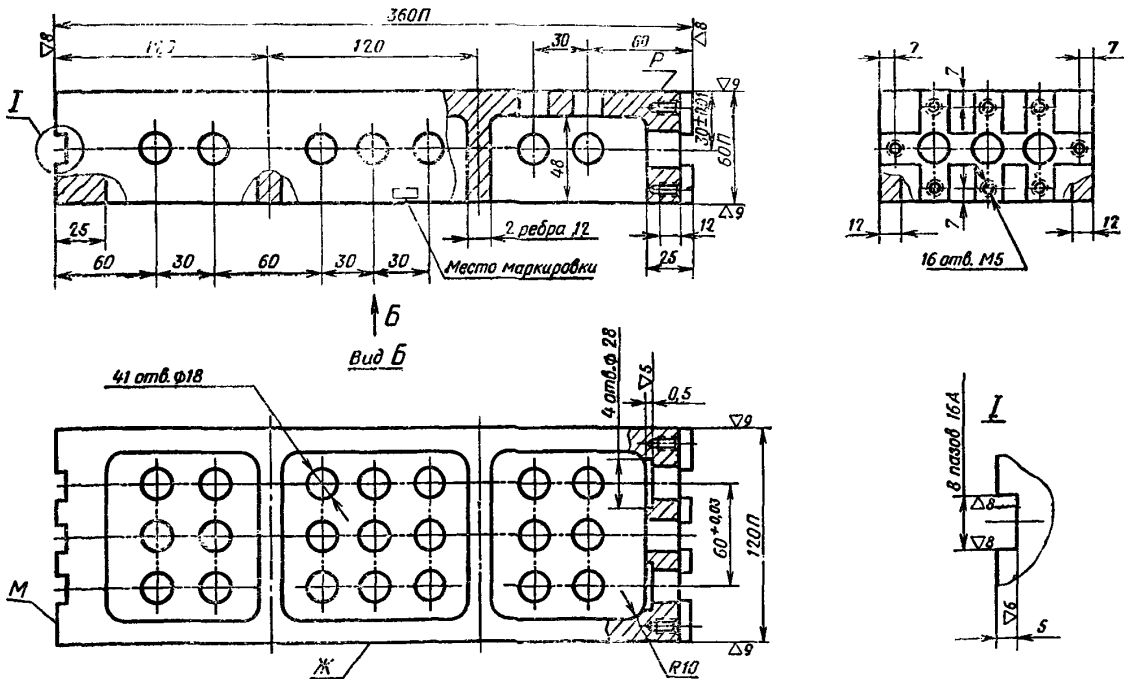
Поверхности М, Ж, Р — базы для контроля.
