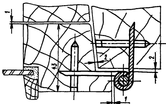
Петля. Тип ПВСм 100 Окно со спаренными переплетами
