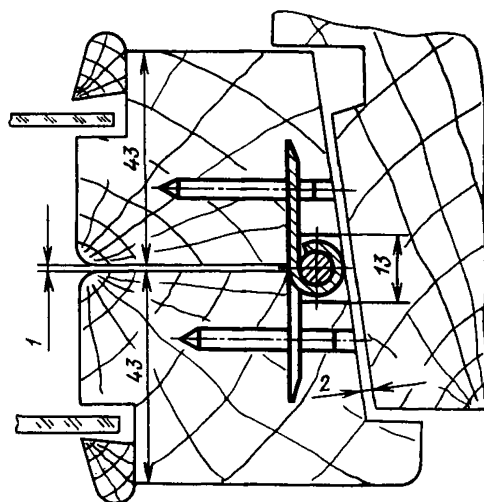
Петля. Тип ПВСм 90 Окно со спаренными переплетами
