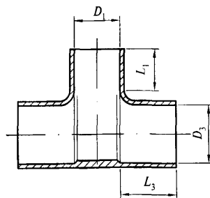
Рисунок Д.6 — Тройник переходный
