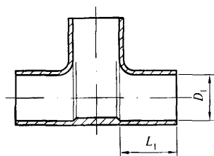
Рисунок Д.5 — Тройник равнопроходный
