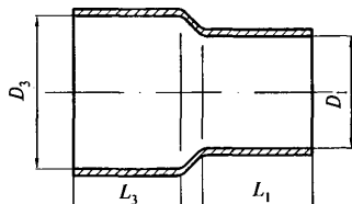
Рисунок Д.3 — Переход
