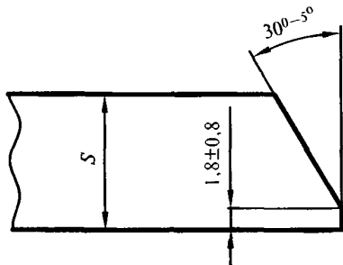
Рисунок 9 — Схема обработки кромок
