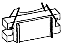
Схема строповки фигурной детали
