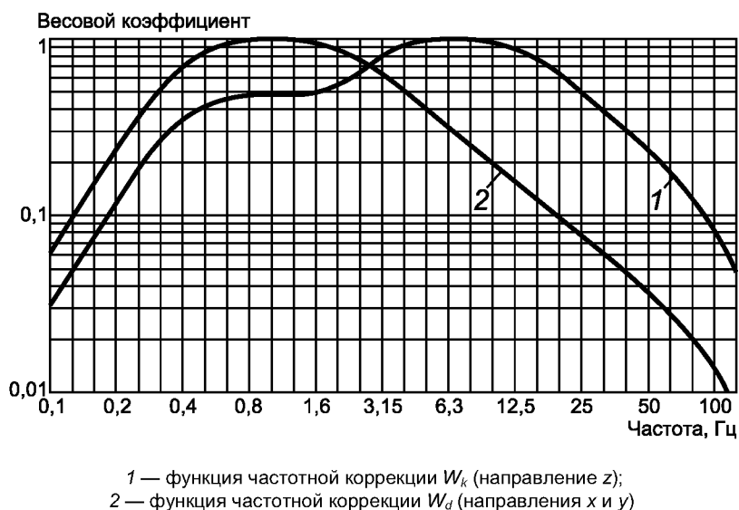
Рисунок В.1 — Функции частотной коррекции W_k и W_d для определения параметров общей вибрации
