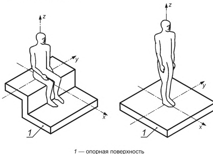
Рисунок 1 — Направления осей базицентральной системы координат
