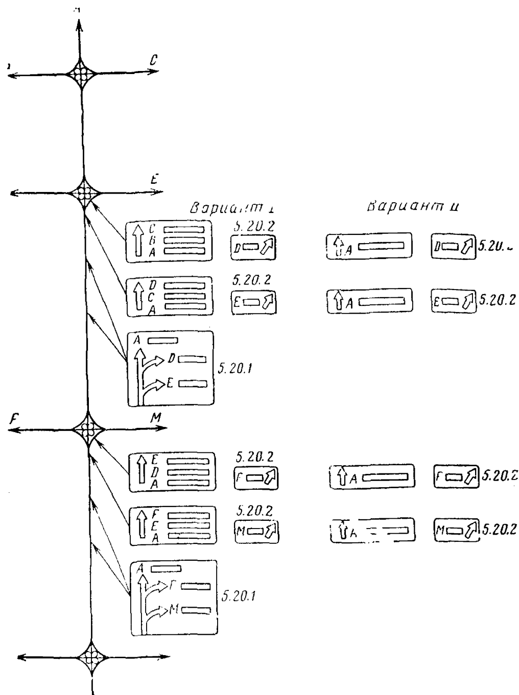
Рис. 11.1. Варианты информации на предварительных указателях направлений движения
