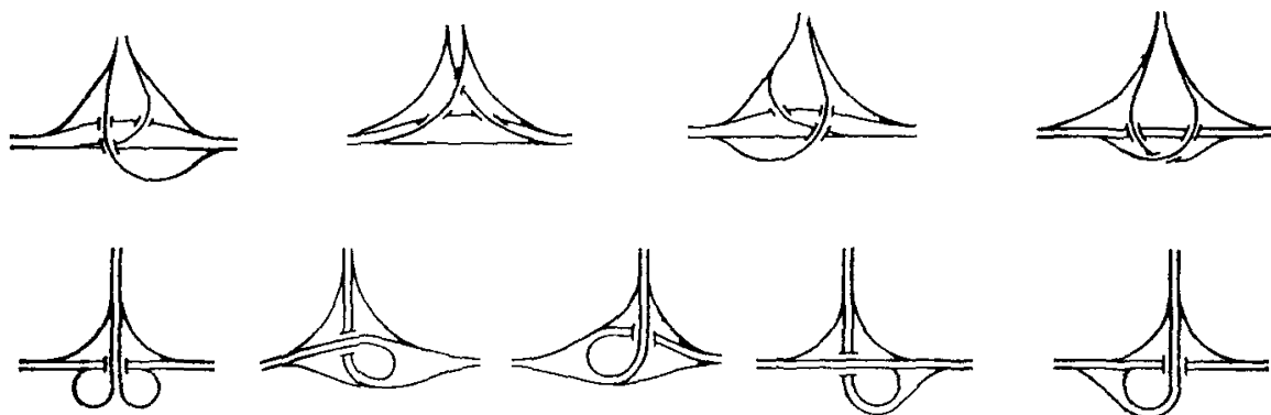
Рис. 8.8. Полные примыкания
