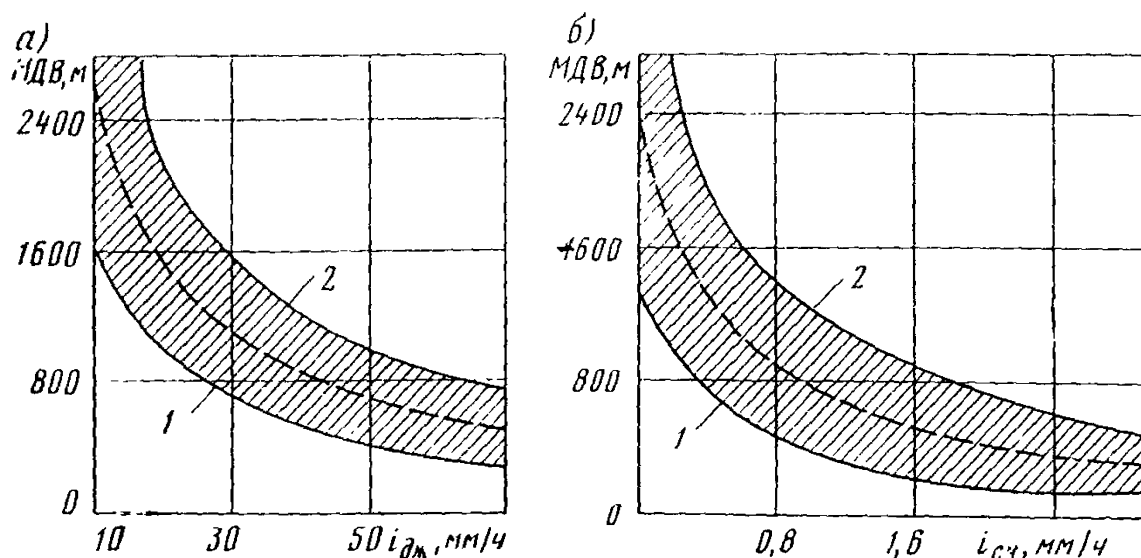
Рис. 6.12. Зависимость метеорологической дальности видимости (МДВ) от интенсивности i_{dj} осадков во время:
