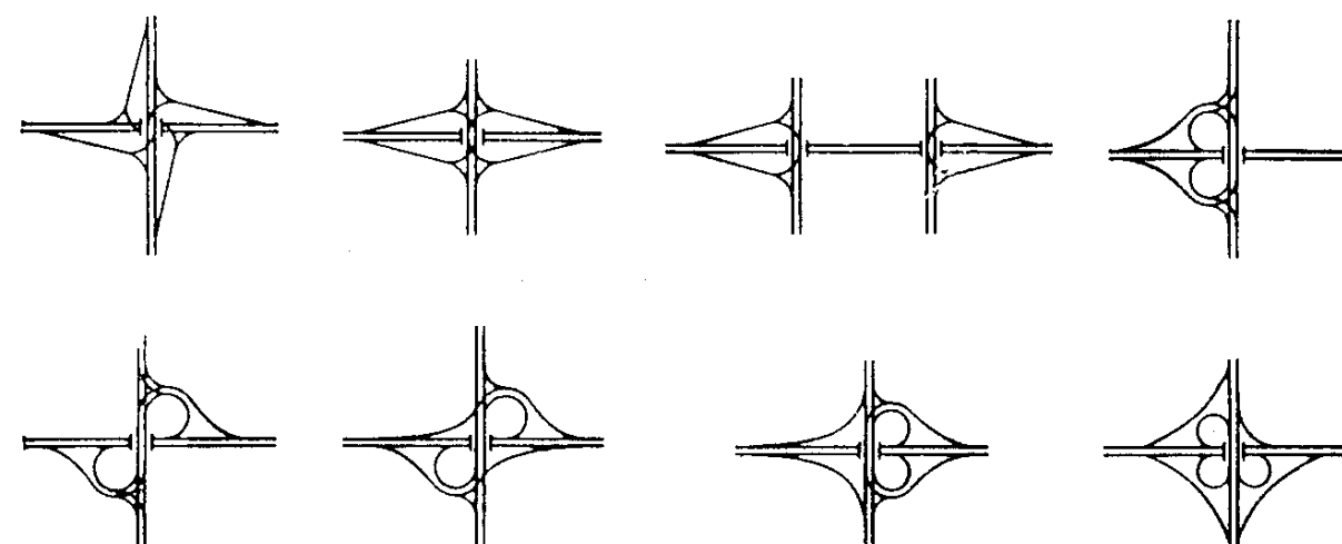
Рис. 8. 2. Неполные пересечения
