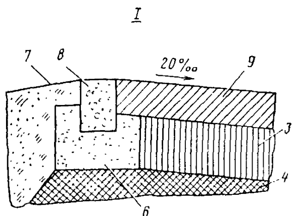
Рис. 7.2. Поперечный профиль в проезжей части с вкопанным бордюром:
