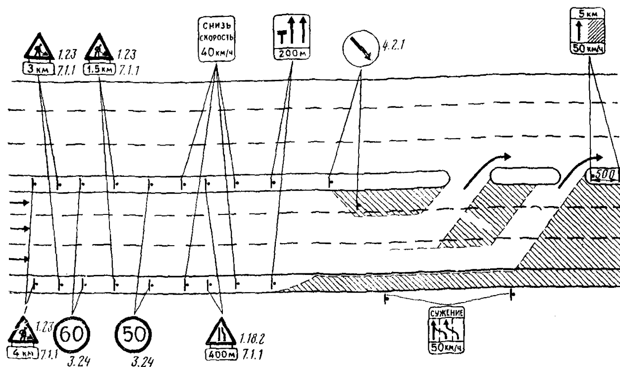
Рис. 10.9. Схема расстановки знаков на подходе к участку ремонтных работ
