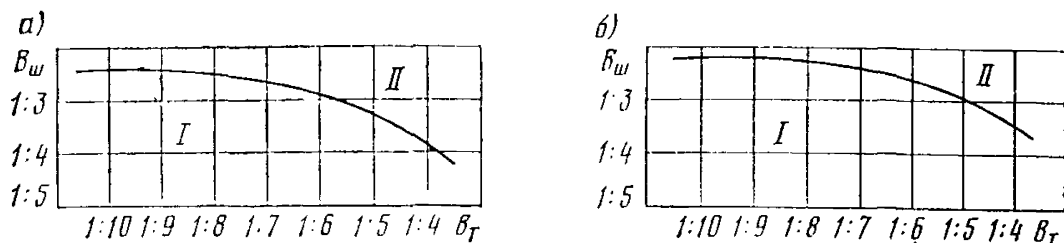
Рис. 7.5. Соотношения заложения внешних B_{ш} и внутренних B_{т} откосов боковых канав треугольной (а) и трапецидальной (б) форм:
