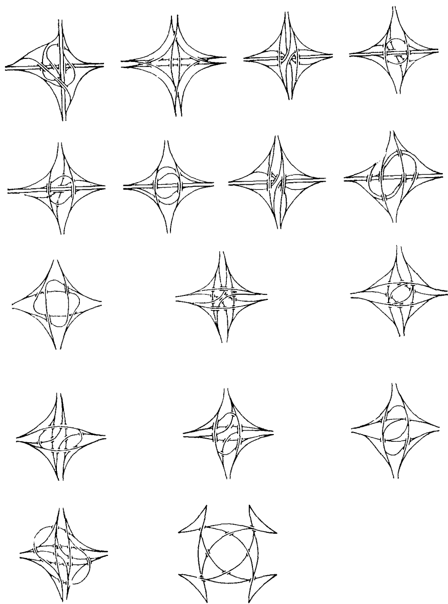
Рис. 8.5. Полные пересечения левоповоротного типа с полупрямыми или прямыми левоповоротными съездами
