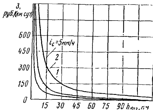
Рис. 6.11. Затраты Z на патрульную снегоочистку в зависимости от допускаемой толщины h_{\text{доп}} слоя рыхлого снега на дороге и интенсивности i_{\text{с}} снегопада
