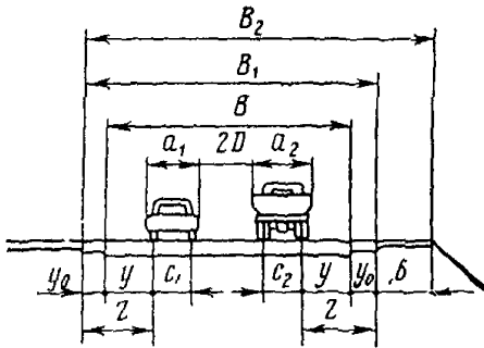
Рис. 6.7. Схема к расчету ширины укрепления поверхности дороги
