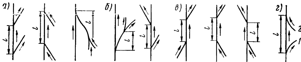
Рис. 8.13. Варианты планировки съездов, определяющие выбор расстояния l между съездами пересечений в разных уровнях
