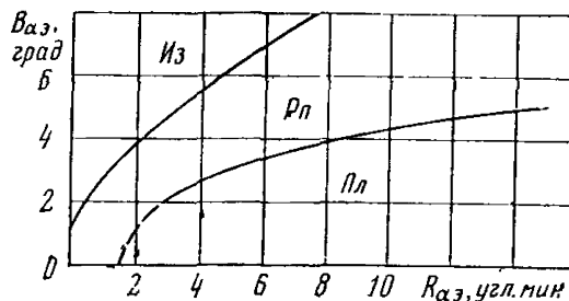
Рис. 5.1. Соотношение кривизны R_{\alpha\epsilon} ведущей линии с видимой шириной B_{a\epsilon} проезжей части в экстремальной точке дороги, обеспечивающих зрительную плавность дороги
