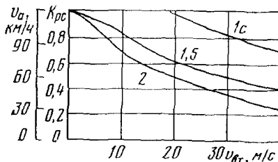
Рис. 6.13. Влияние скорости ветра v_{\text{вт}} на обеспеченность расчетной скорости v_{\text{а}} при времени реакции водителя 1, 1,5 и 2 с
